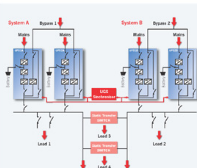
Конфигурация dynamic dual bus
