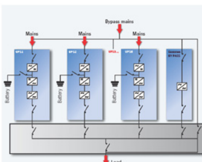
Параллельная конфигурация до 8 ИБП при общем байпасе
