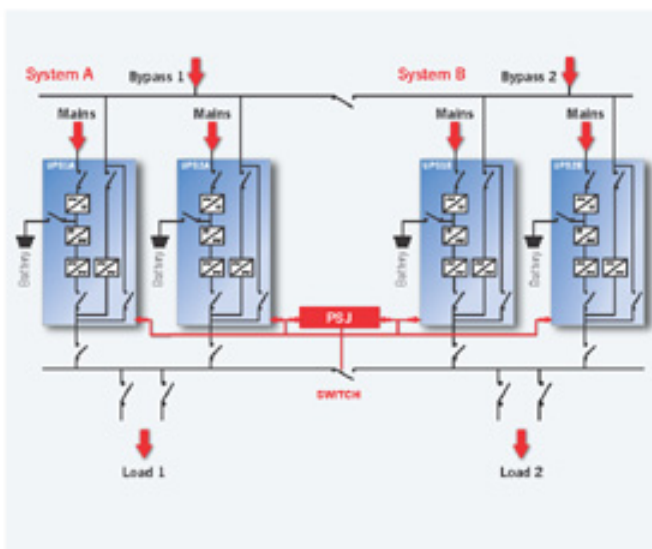
Конфигурация dual bus system
