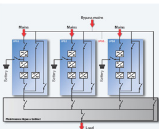
Параллельная конфигурация до 8 ИБП при распределенном байпасе
