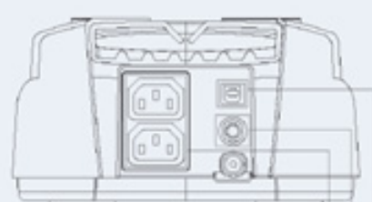
РОЗЕТКИ IEC ПОД ЗАЩИТОЙ ИБП ЗАЩИТНЫЙ ПРЕДОХРАНИТЕЛЬ USB-ПОРТ ДЛЯ ОБМЕНА ИНФОРМАЦИЕЙ
